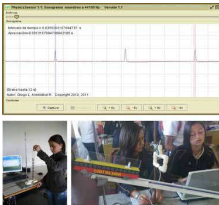
Figura 18. Sonoscopio (arriba) y aplicaciones de la Fotocpuerta (abajo) de PhysicsSensor
