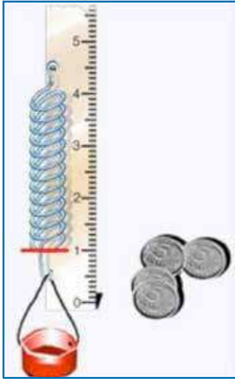
Figura 1.1. El peso de un cuerpo puede determinarse por medio de un dinamómetro o balanza de resorte.
